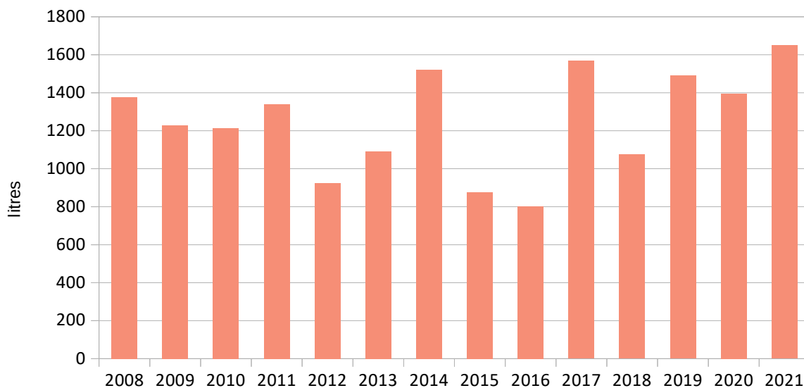
Gràfic 1. Comparativa del consum de combustible entre els anys 2008 i 2021.
