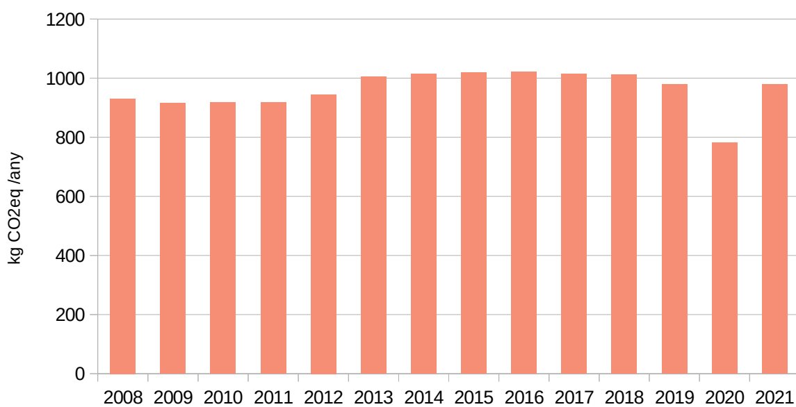
Gràfic 8. Comparativa de les emissions per treballador a causa dels desplaçaments al centre de treball dels anys 2008 a 2021.
