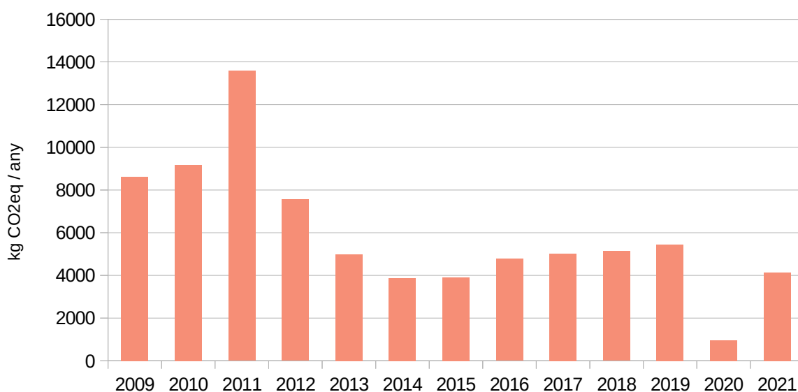
Gràfic 10. Comparativa de les emissions per mobilitat dels assistents a cursos i jornades. CEACV entre 2009 i 2021.
