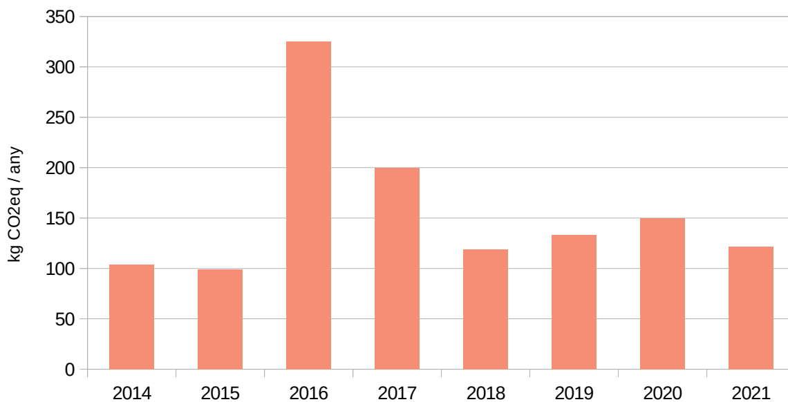
Gràfic 12 . Comparativa de les emissions pel consum d'aigua entre 2014 i 2021.
