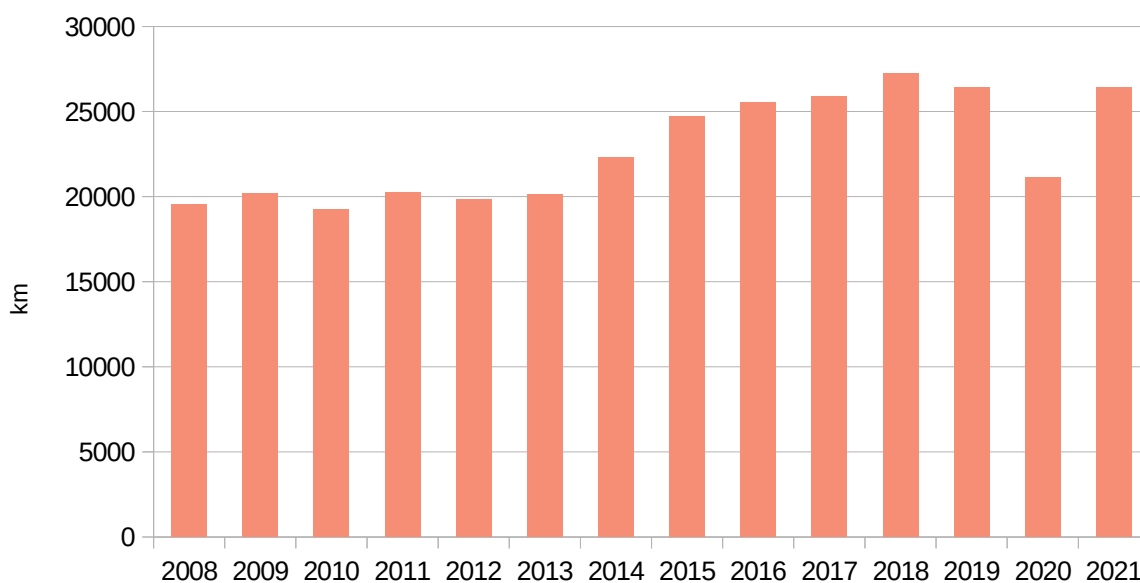
Gràfic 7. Comparativa de les emissions degudes al transport del personal al centre de treball en vehicles privats entre els anys 2008 a 2021.
