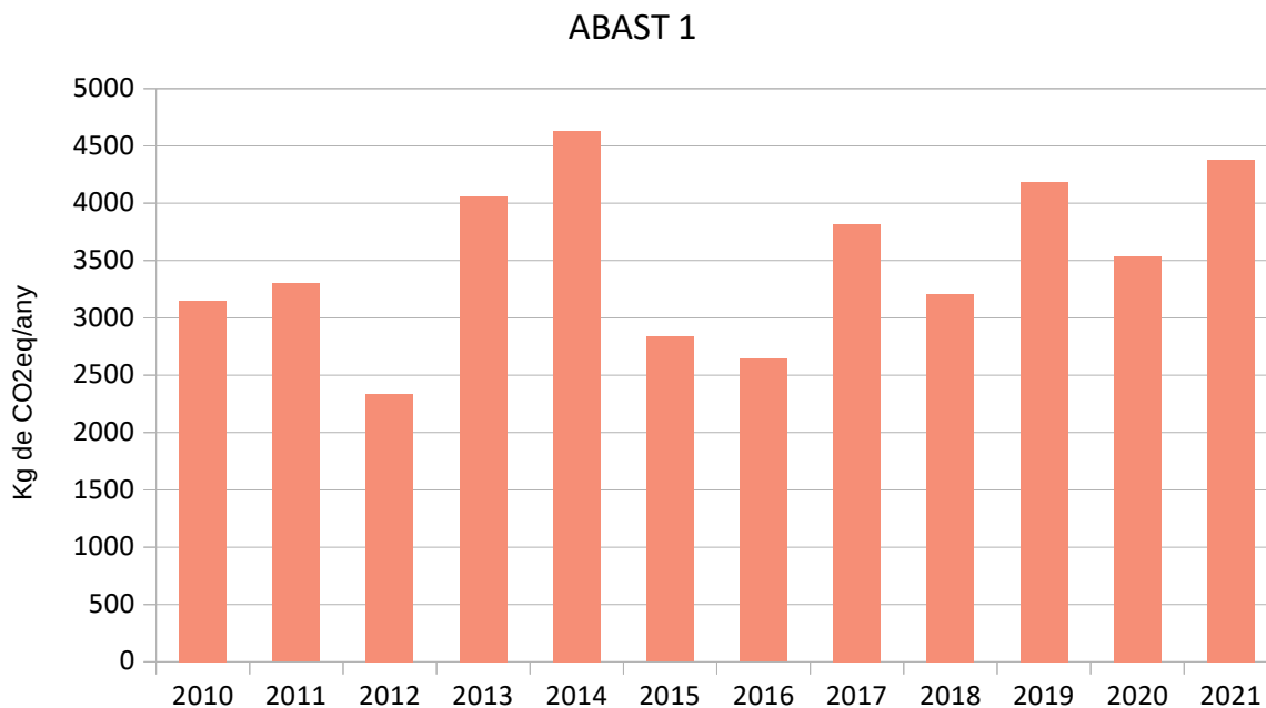
Gràfic 3. Comparativa de les emissions ABAST 1 de 2010 a 2021.
