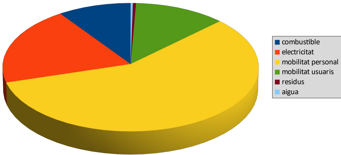
Gràfic 14. Emissions totals diferenciades per activitats 2021.
