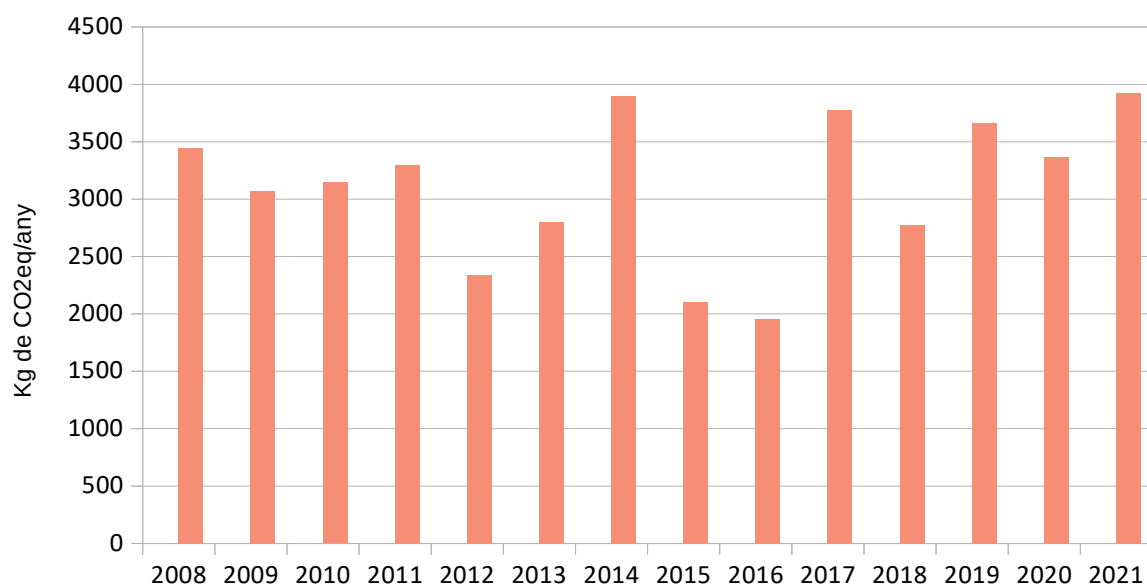
Gràfic 2. Comparativa de les emissions degudes al consum de combustible entre els anys 2008 i 2021
