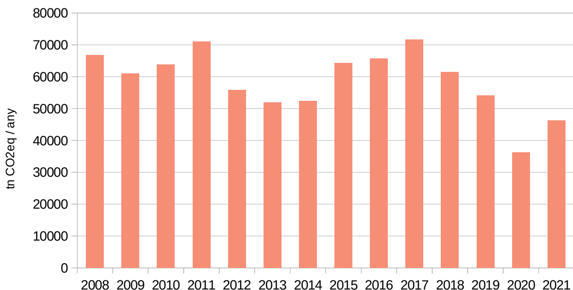
Gràfic 13. Comparativa de les emissions totals generades per les activitats del CEACV de 2008 a 2021.
