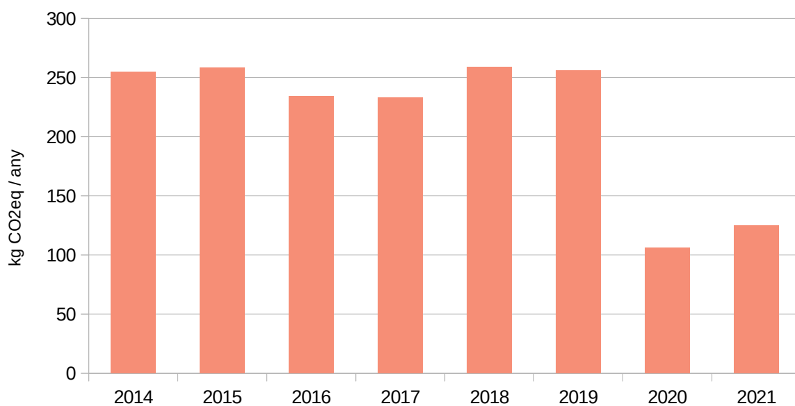
Gràfic 11. Comparativa de les emissions per generació de residus urbans, entre 2014 i 2021.
