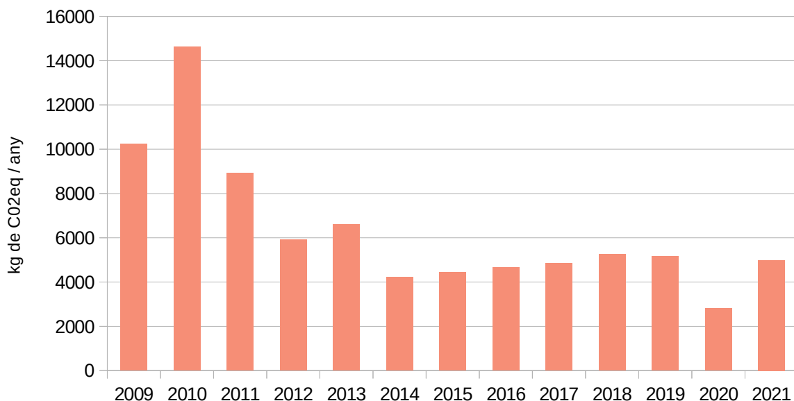
Gràfic 9. Comparativa de les emissions per la mobilitat dels grups que van visitar el CEACV, entre 2009 i 2021.
